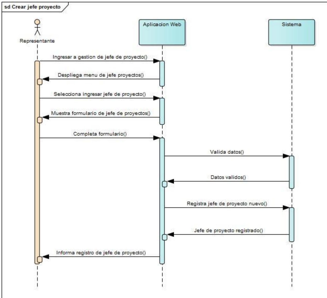
Ilustración 30 Diagrama de secuencia Crear jefe de proyecto
