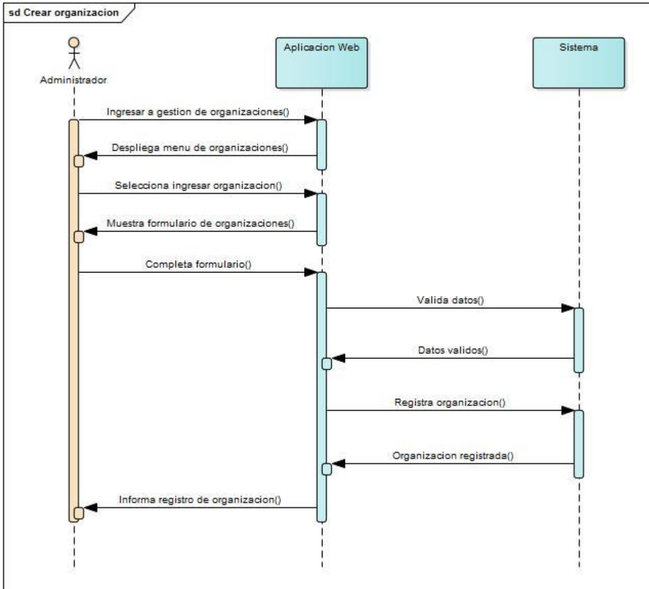
Ilustración 34 Diagrama de secuencia Administrador Crear organización
