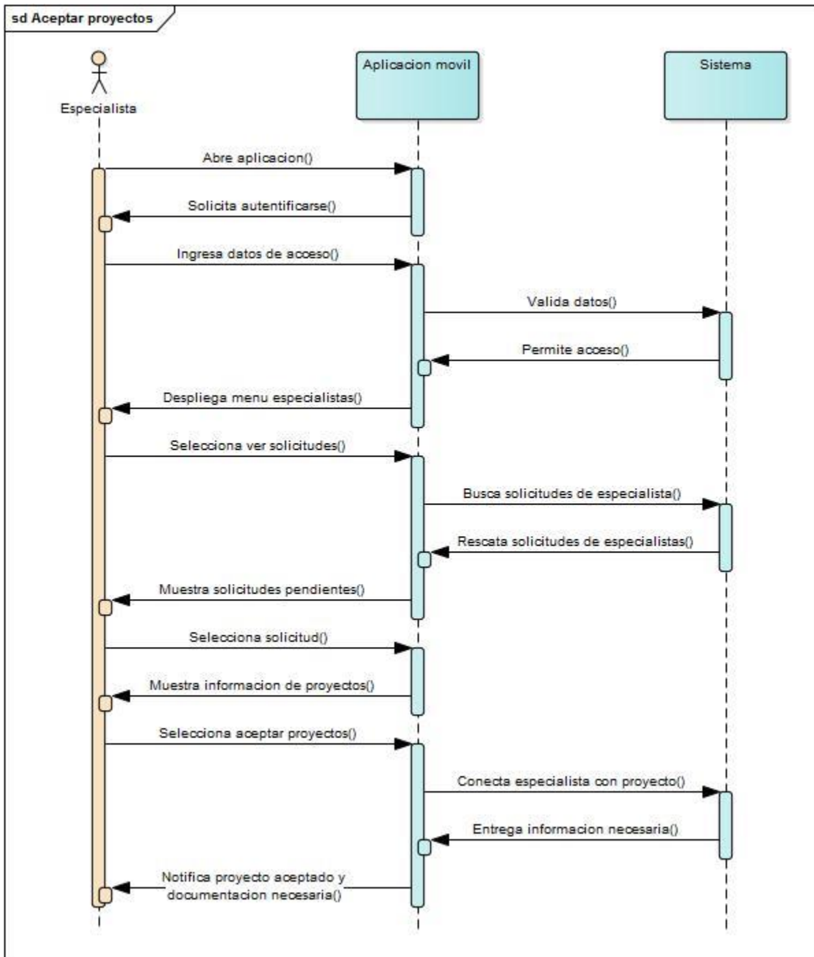
Ilustración 32 Diagrama de secuencia Especialista Aceptar proyectos
