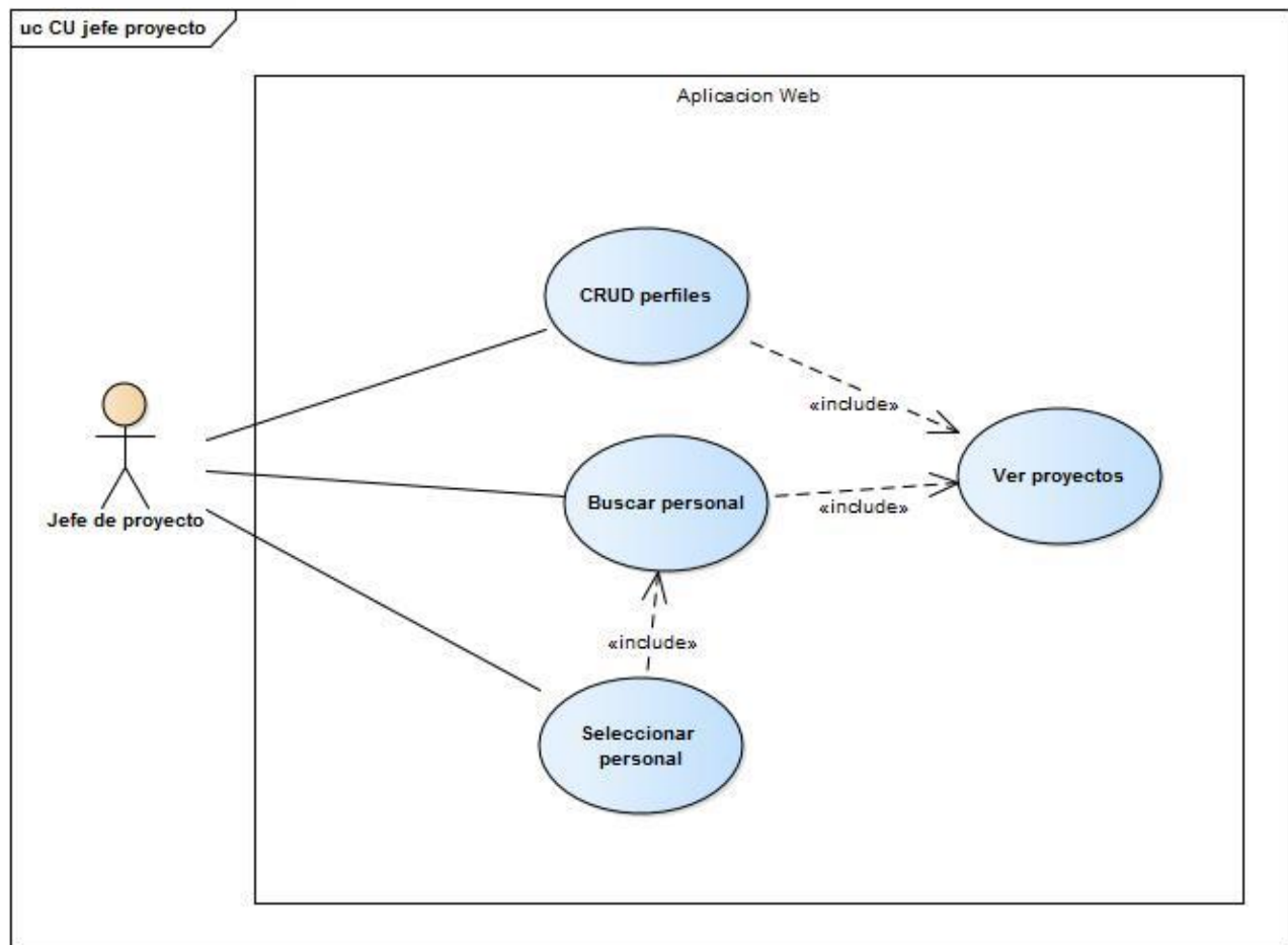
Ilustración 14: Caso de uso de Jefe de proyecto
