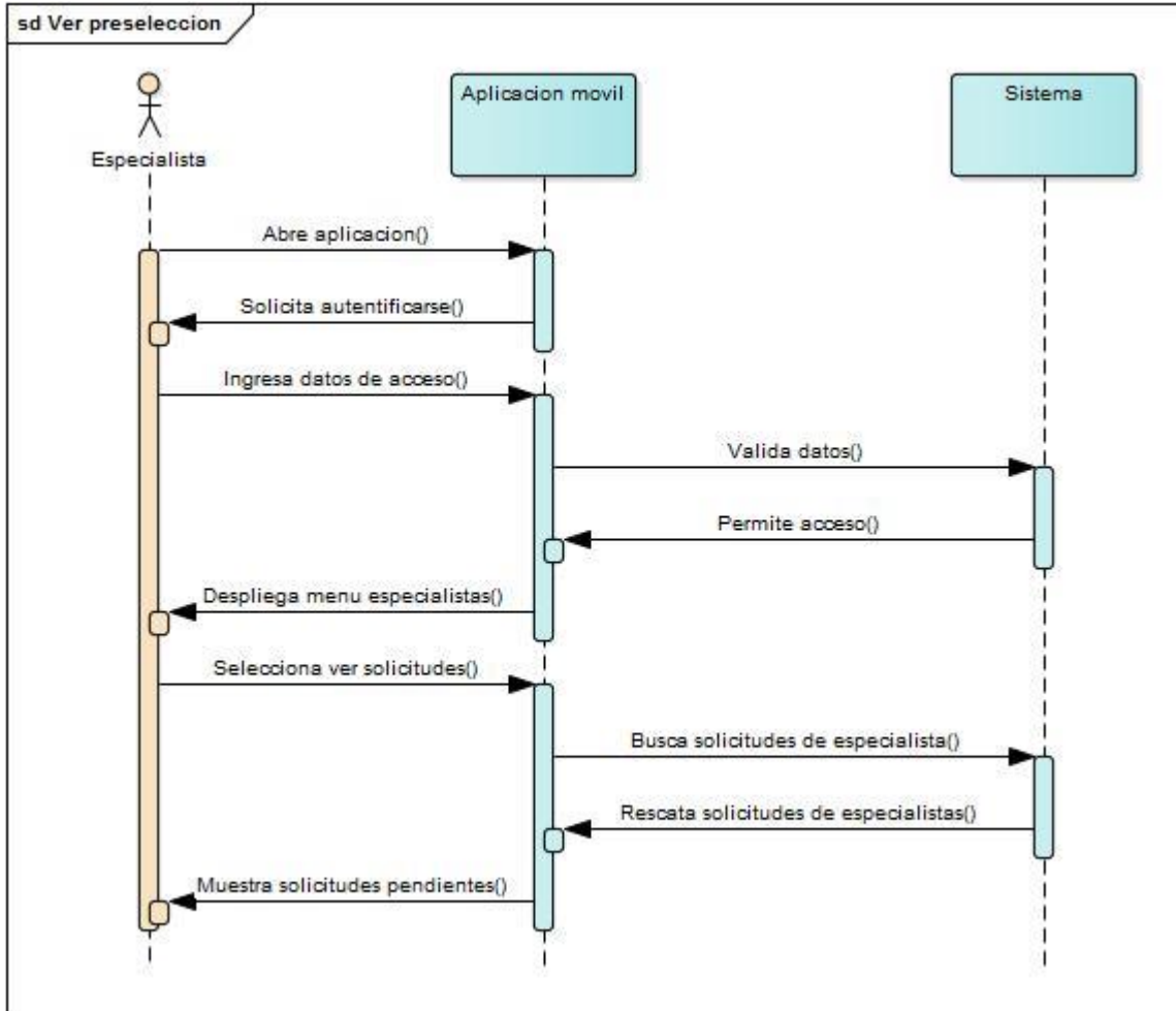
Ilustración 31 Diagrama de secuencia Especialista Ver preselección
