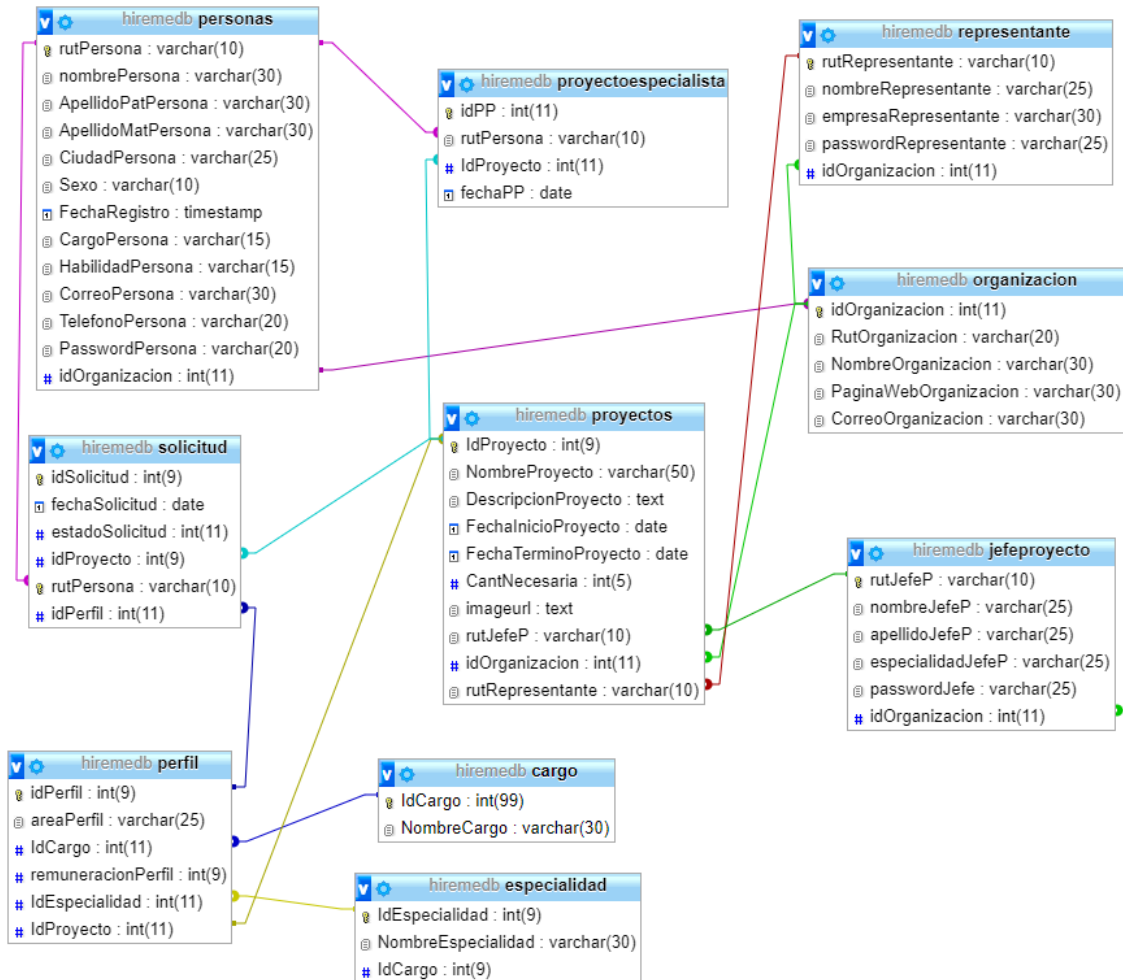
Ilustración 24: Modelo de datos
