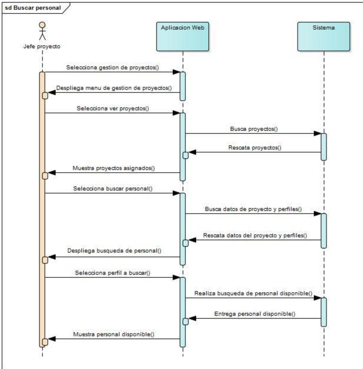
Ilustración 28 Diagrama de secuencia Buscar personal
