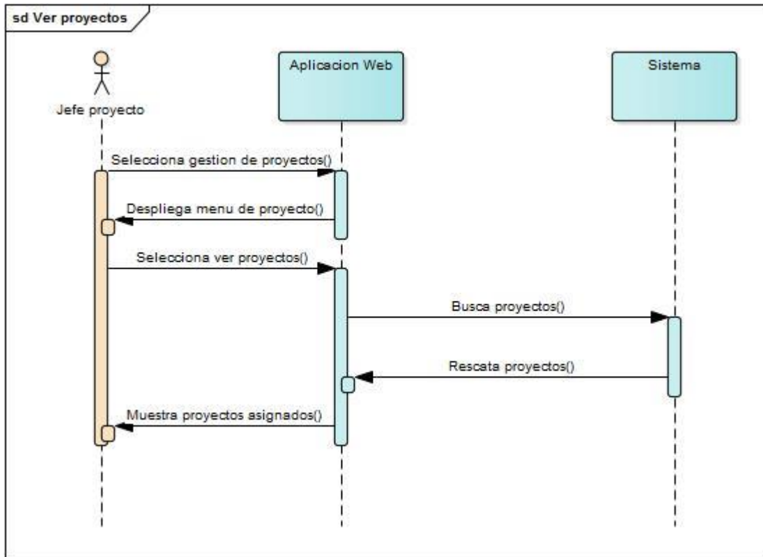
Ilustración 25 Diagrama de secuencia ver proyectos
