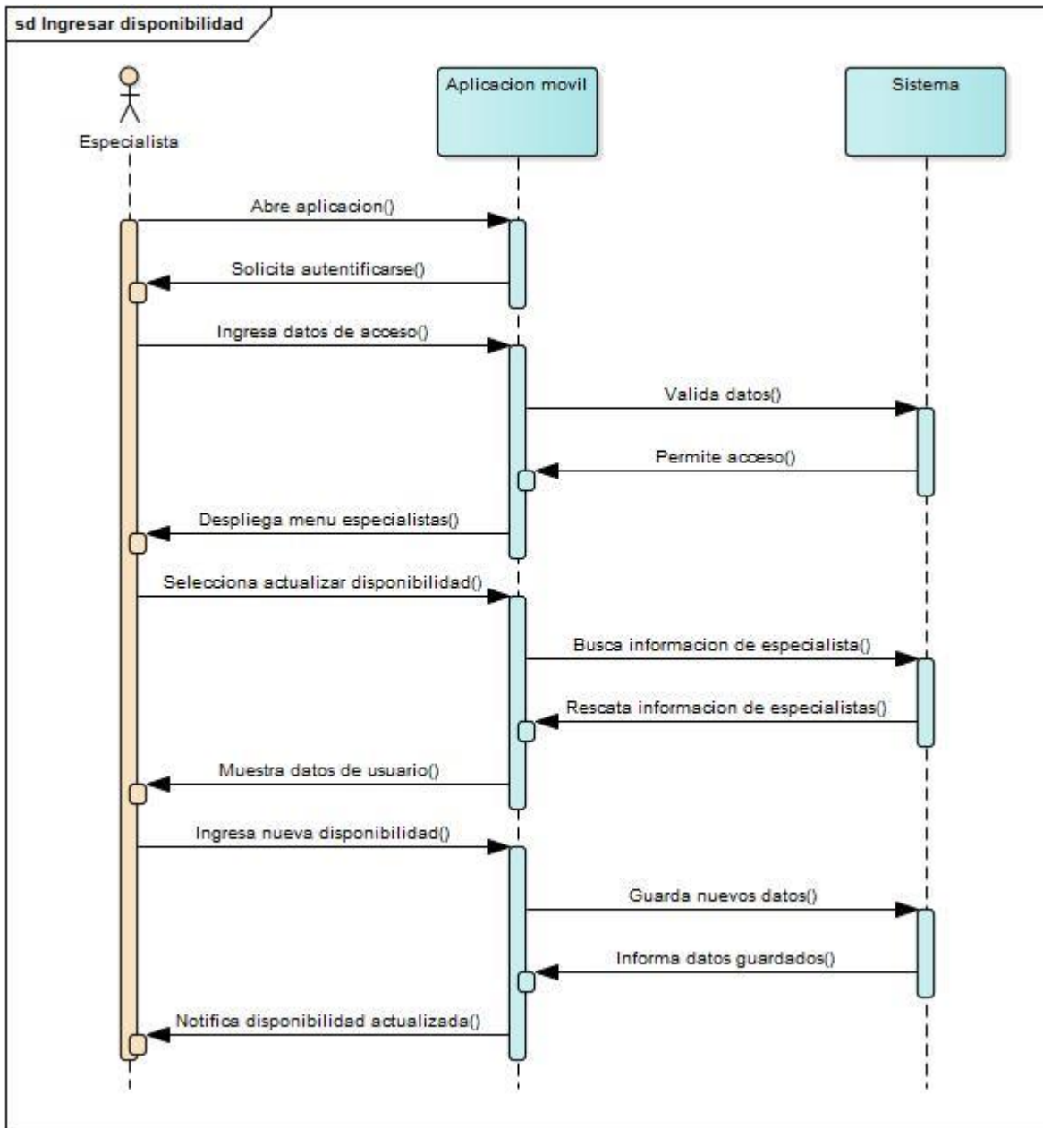
Ilustración 33 Diagrama de secuencia Ingresar disponibilidad
