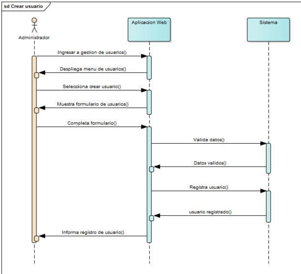
Ilustración 35 Diagrama de secuencia Crear Usuario
