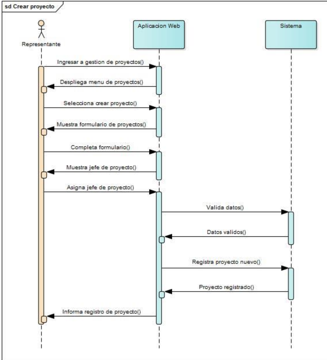
Ilustración 29 Diagrama de secuencia representante crear proyecto
