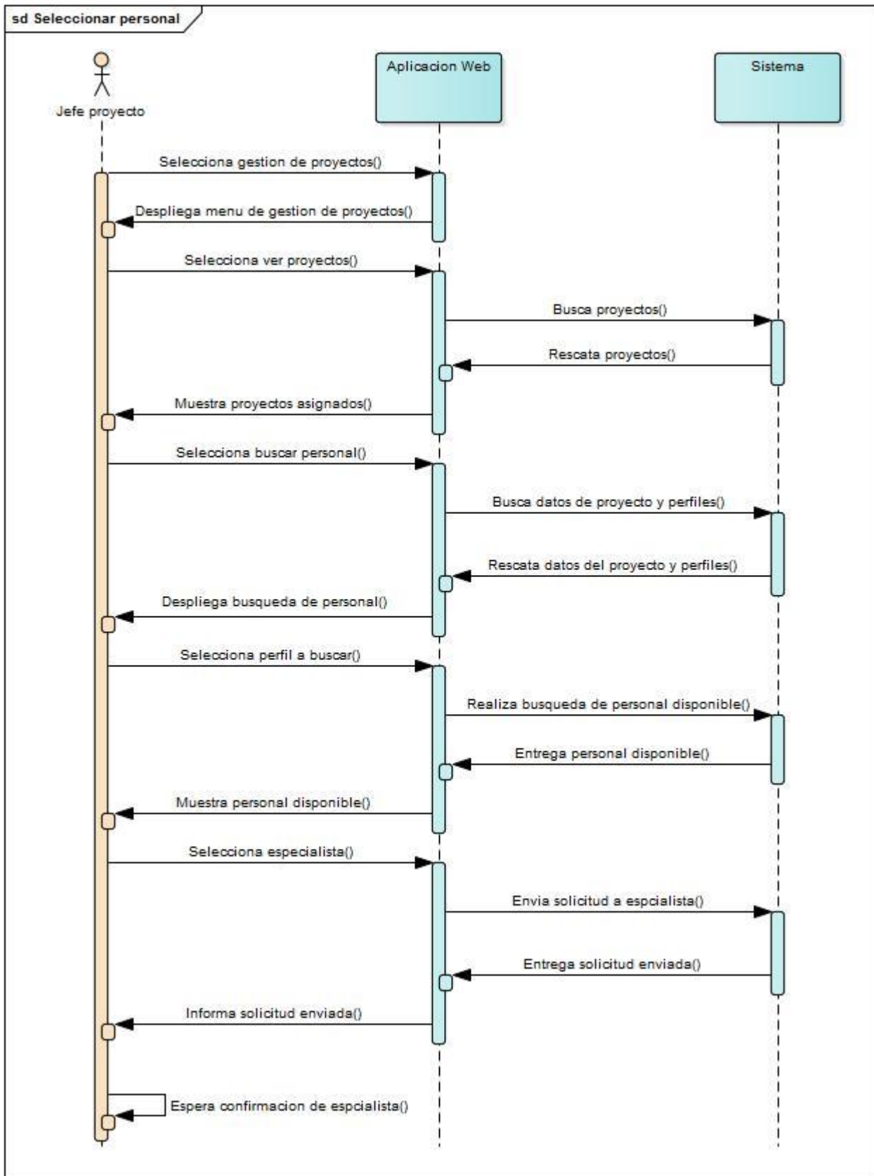
Ilustración 26 Diagrama de secuencia Seleccionar personal
