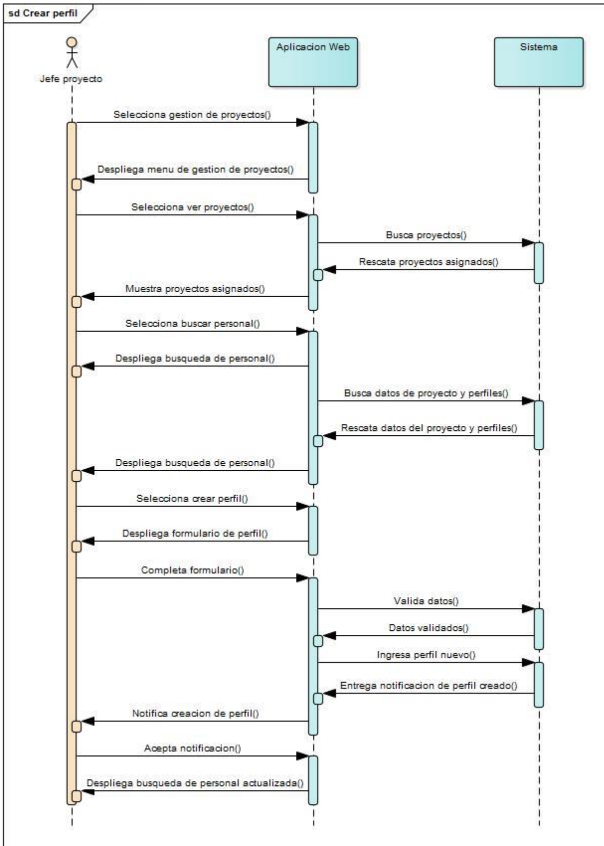
Ilustración 27 Diagrama de secuencia Crear perfil
