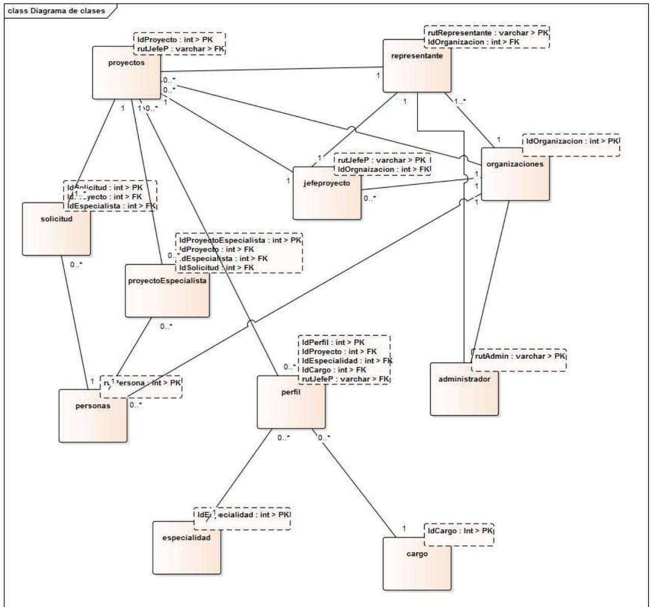
Ilustración 23: Diagrama de clases
